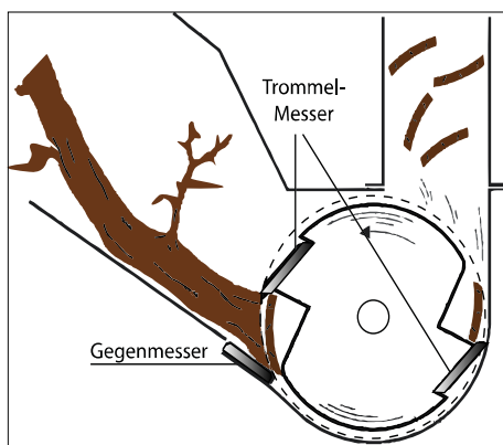
Duplex-Messertrommel
